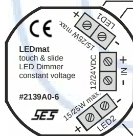
Ansicht Baugruppe / board view
